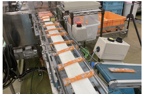
長い包材にゼリー液を充填した後、1本ずつカットする。
